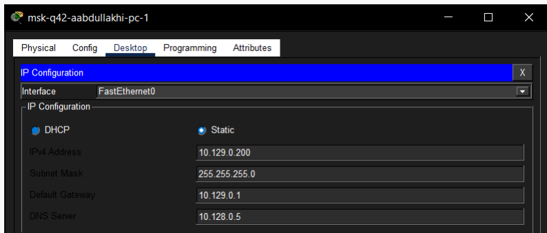
Рис. 8: Настройка IP-адреса на ПК сети 42-го квартала
