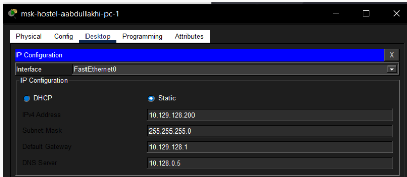
Рис. 11: Настройка IP-адреса на ПК сети общежития
